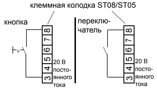
Клеммы 3/8 для подключения цифрового входа - системная плата (клеммная колодка ST08) - плата расширения / релейная плата (клеммная колодка ST05)
